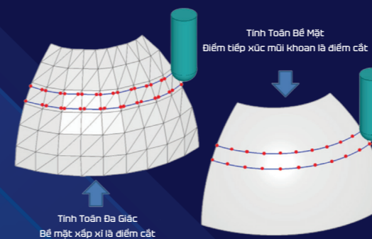
CAM-TOOL sở hữu phương pháp tính toán đường chạy dao ưu việt
